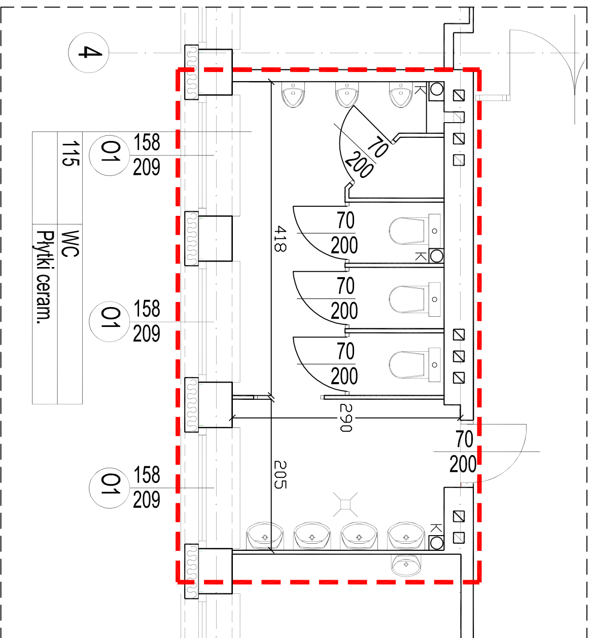
Rzut sanitariatu
