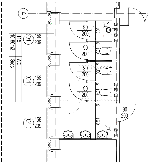
Rzut sanitariatu
