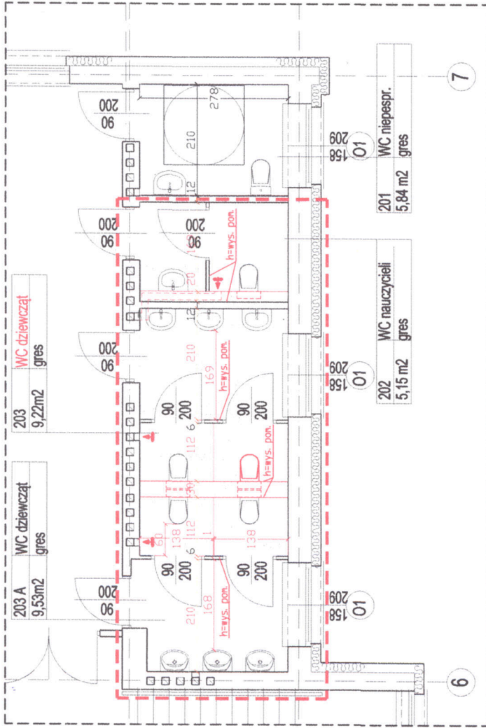
Rzut sanitariatu
